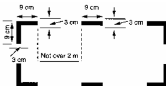
Слика 1 Обележавање места за продор
