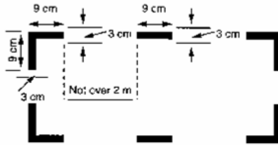
Слика 1 Обележавање тачака за пробијање оплате авиона
