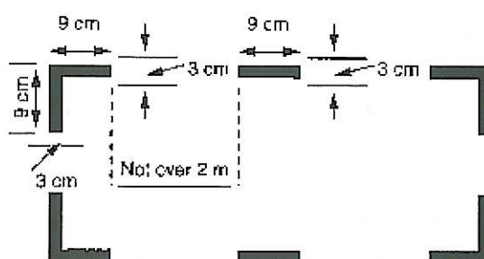
Слика 1 Означивање места за продор
